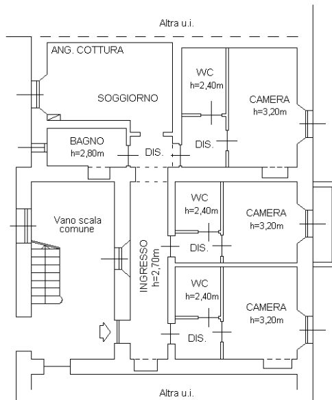
PIANO PRIMO
